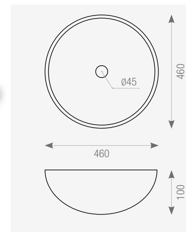
185419 Lavabo Redondo Silver 46x46x10 cm./18.1"x18.1"x3.9" E200
