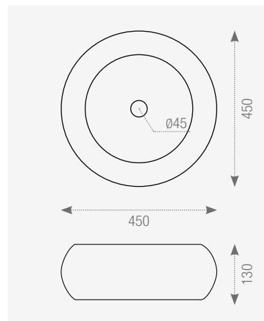
187323 Lavabo Madison 45x45x13 cm./17.7"x17.7"x5.1" E450
